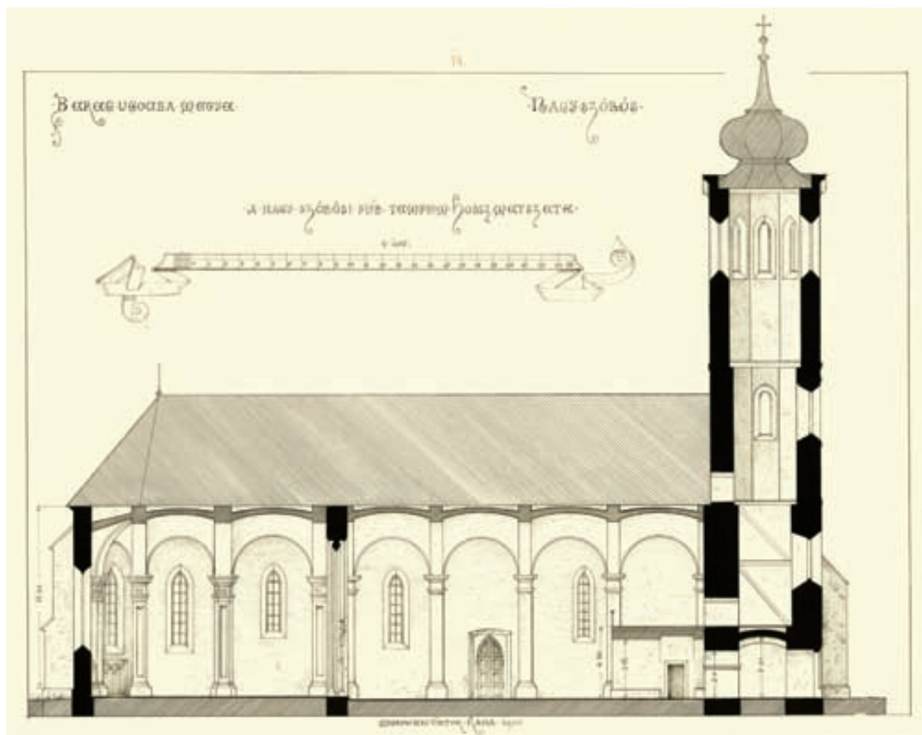
5. A templom hosszmetsete (Myskovszky Viktor, 1900)
