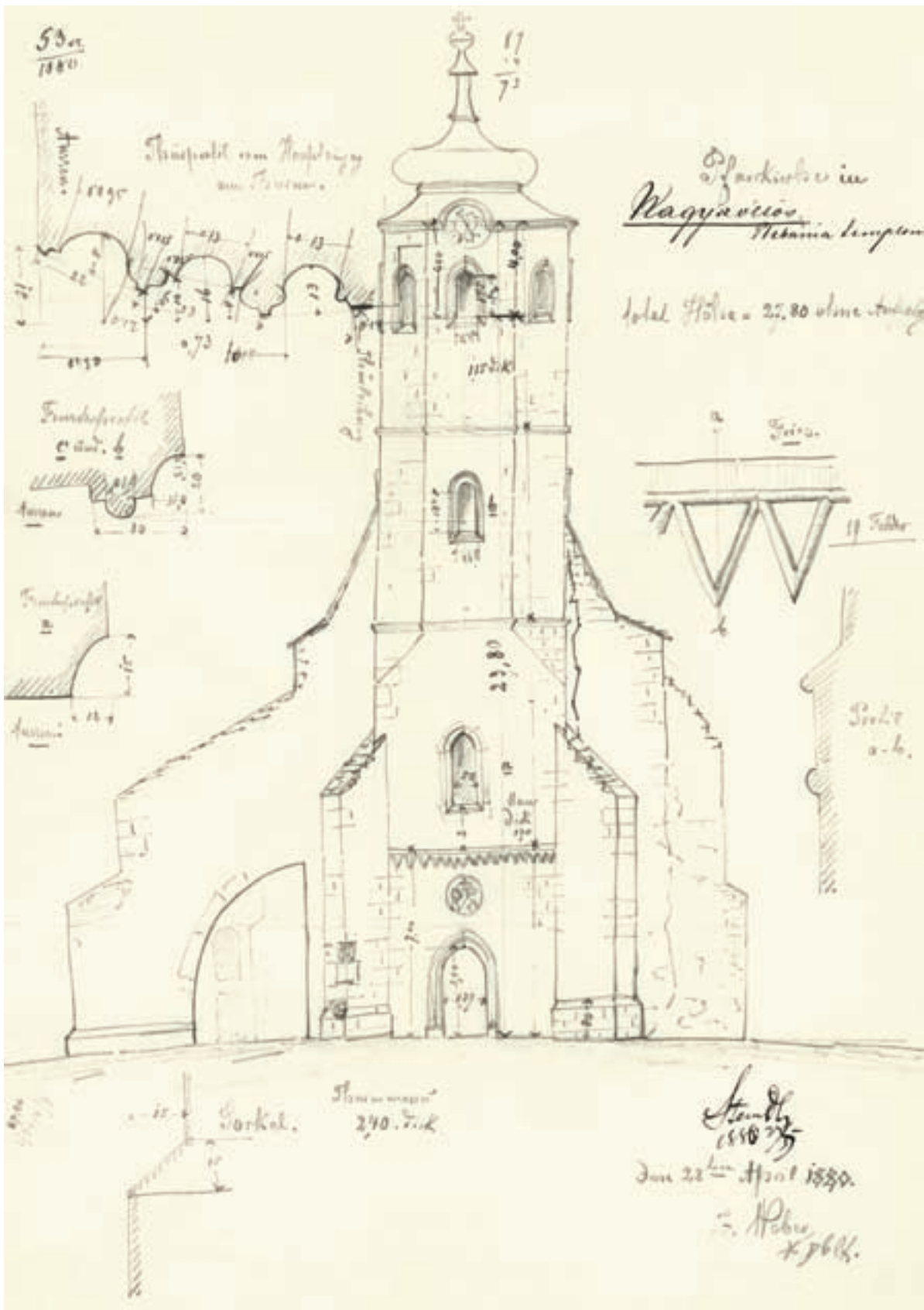
8. A templom nyugati homlokzata részletrajzokkal (Weber J., 1880)
