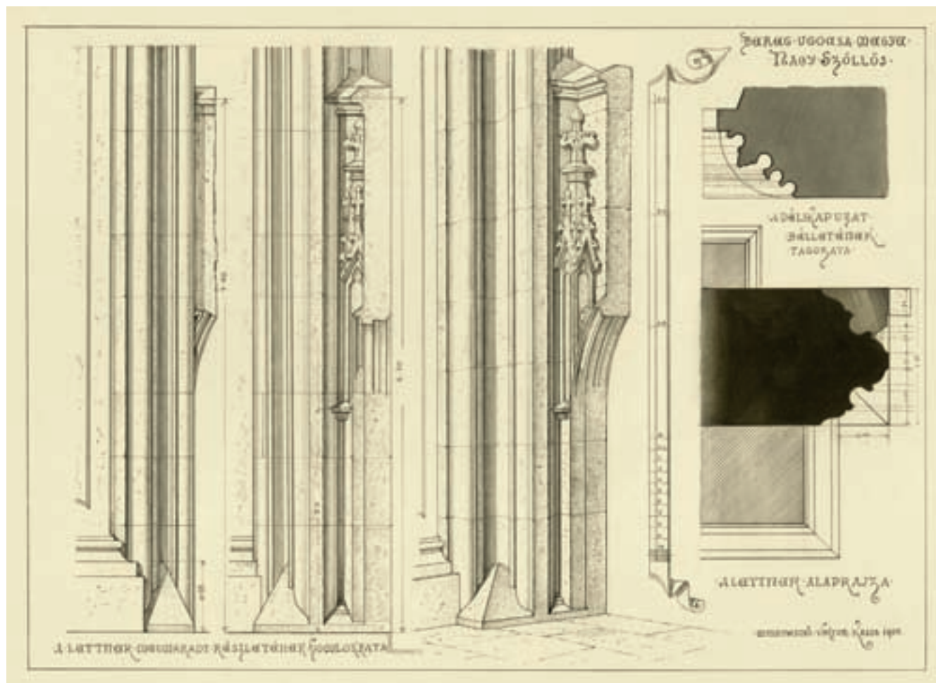
16. Felmérések a lettner megmaradt részéről (Myskovszky Viktor, 1900)
