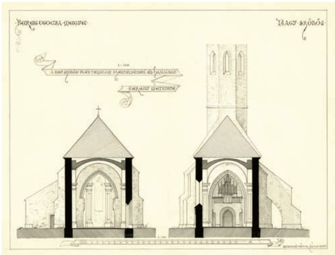
6. A hajó és a szentély keresztmetszete (Myskovszky Viktor, 1900)
