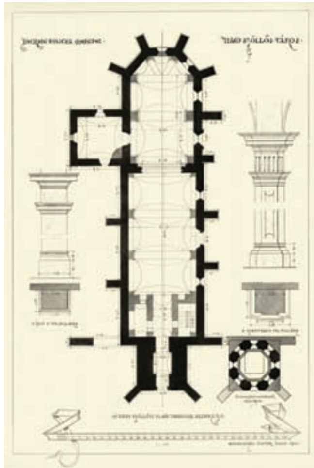
3. A templom alaprajza részletrajzokkal (Myskovszky Viktor, 1900)
