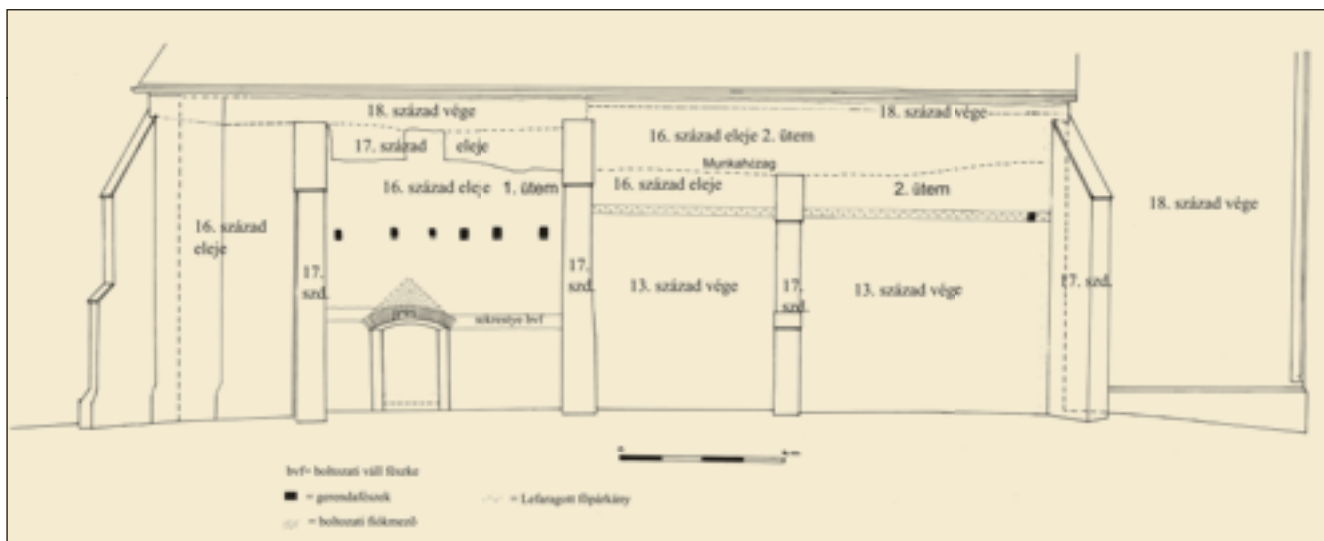
4. A templom északi homlokzatának kutatási felmérése
