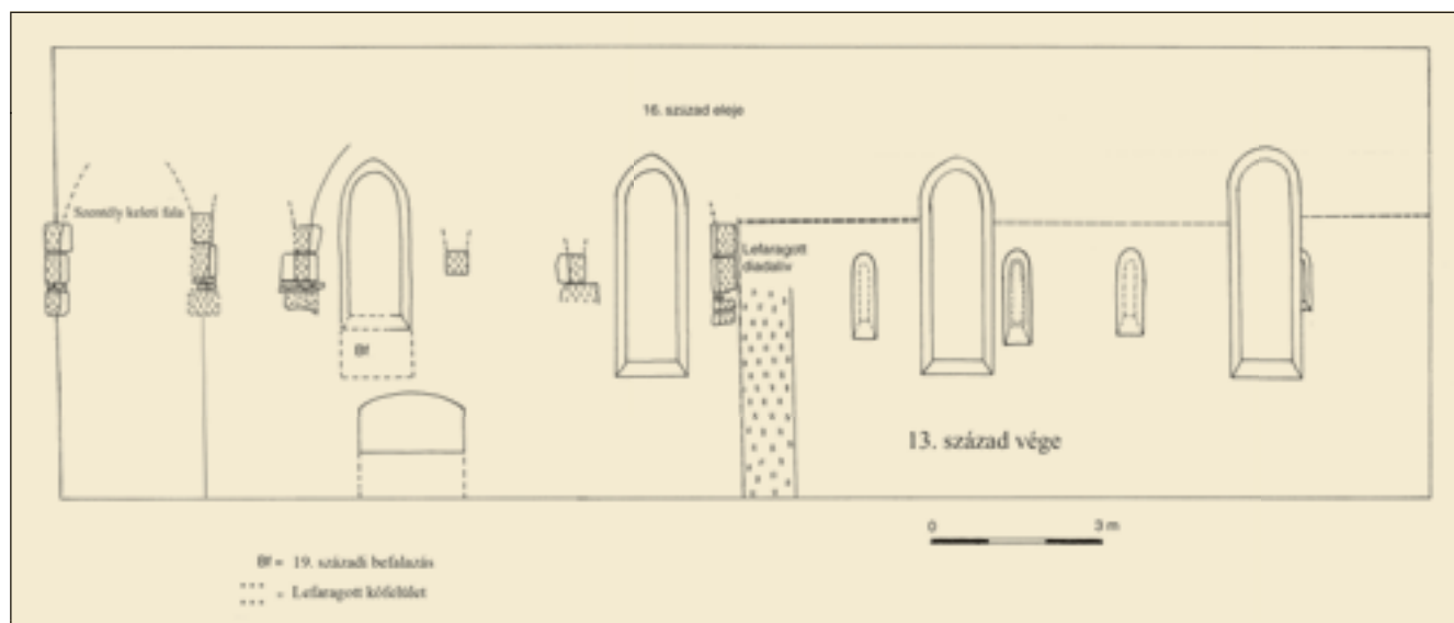
3. A templom déli belső oldalfalának kutatási felmérése
