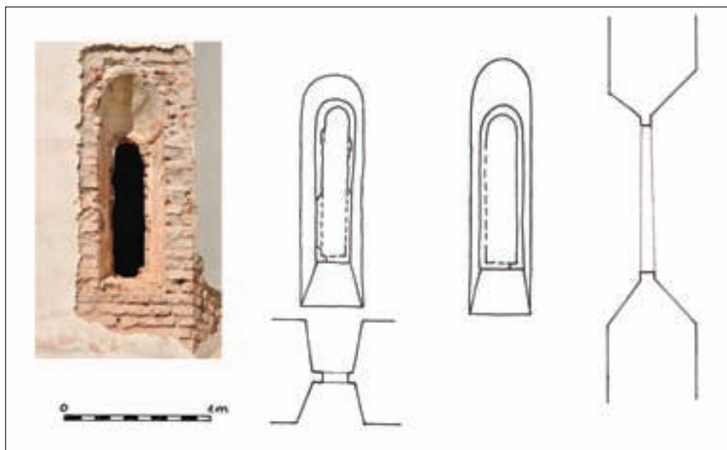
6. A hajó déli falában feltárt román kori ablaknyílás
